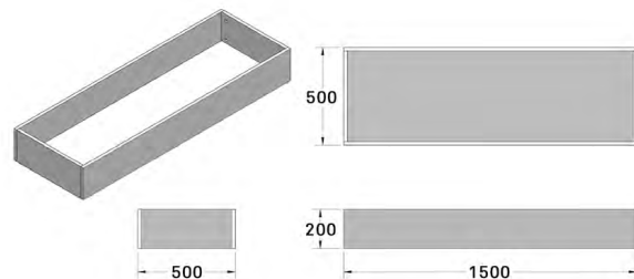
SMP-15 1500 W
